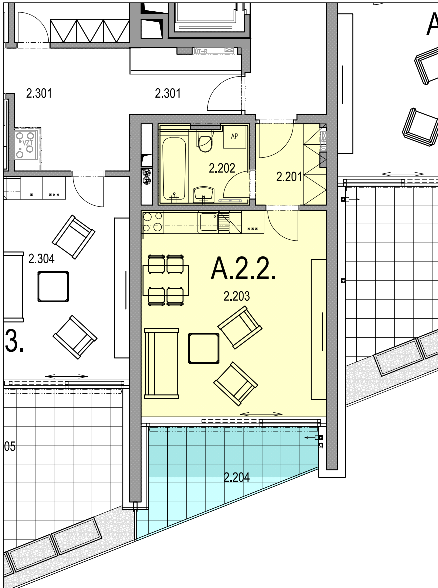
PŮDORYS 2.NP SCHEMA SEKCE A
