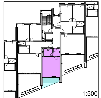
PŮDORYS 2.NP SCHEMA SEKCE B
