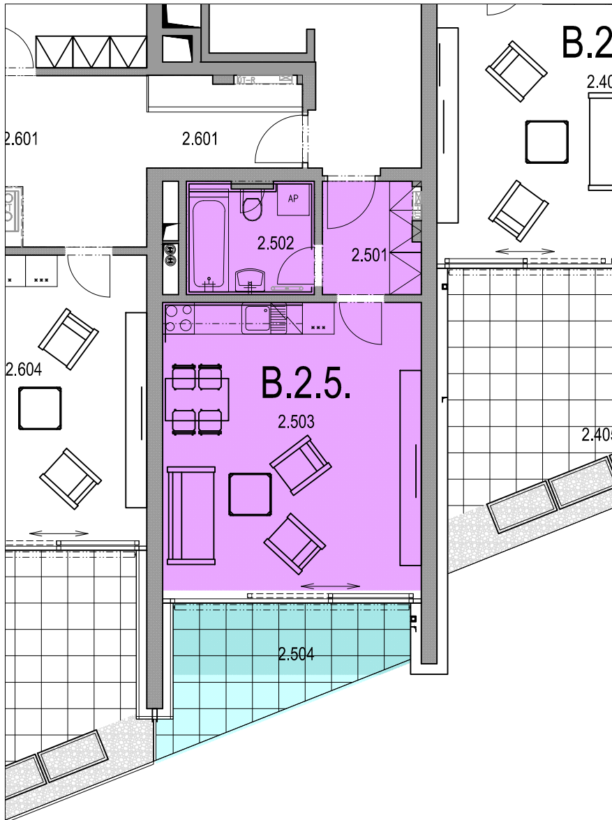
PŮDORYS 2.NP SCHEMA SEKCE B
